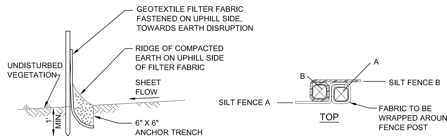
SECTION A-A
